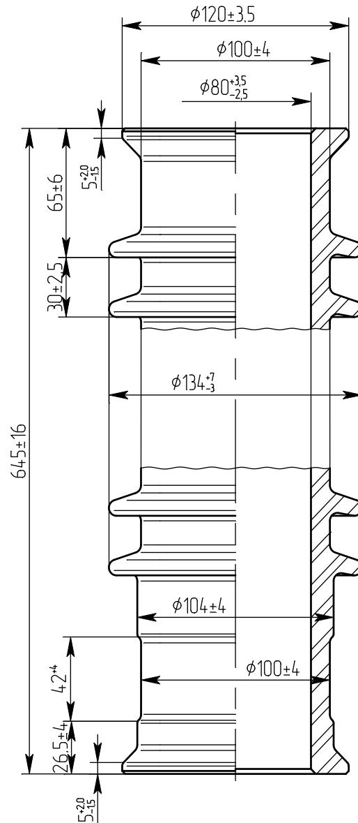
П 645/80 О чертёж НИЮД.703 креслення
