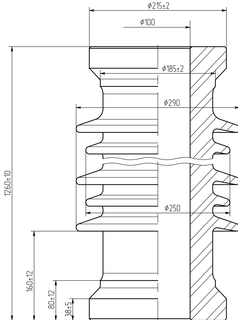
ППН - 1260/100 О чертёж НИЮД.757523.073 креслення
